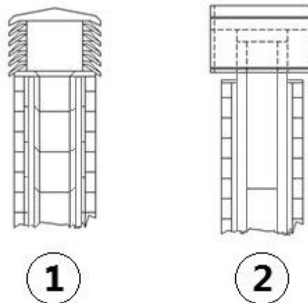
Fig. 4 - Extremos de chimenea antiviento
