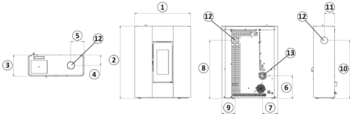
Fig. 19 - Dimensiones generales: Roxy
