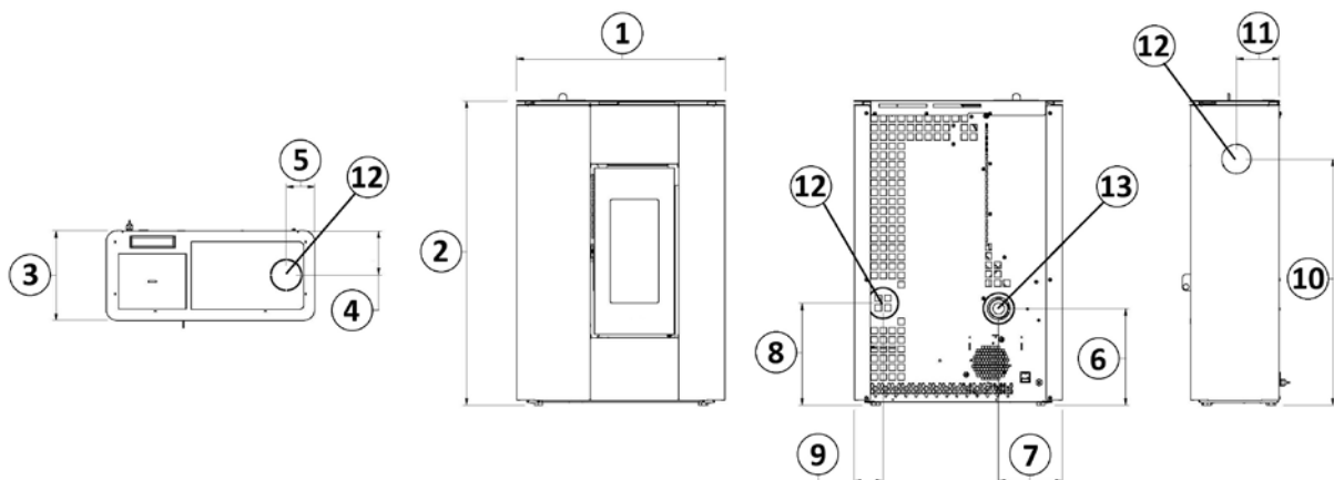
Fig. 18 - Dimensiones generales: Atrium
