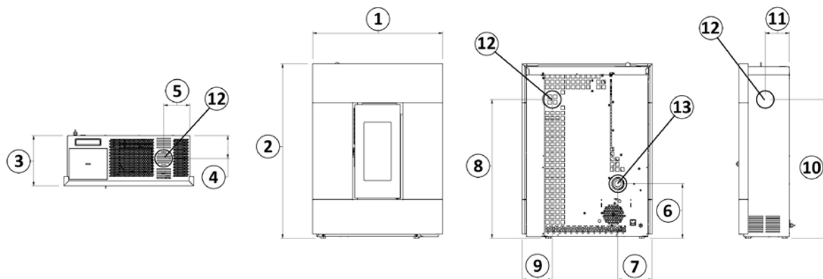
Fig. 21 - Dimensiones generales: Tabla
