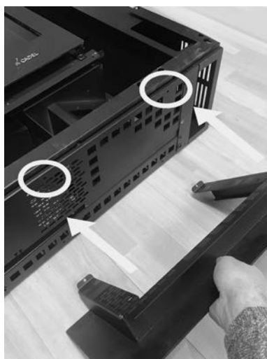
Fig. 48 - Coloque el pedestal
