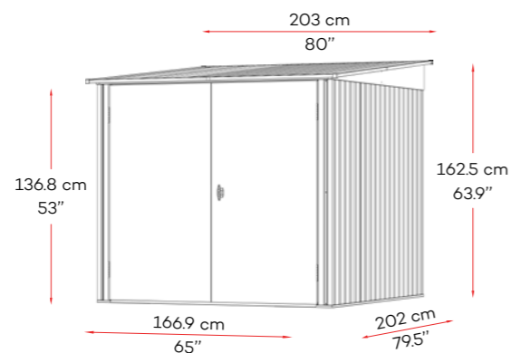
Guarda bicicletas 6'x6'
