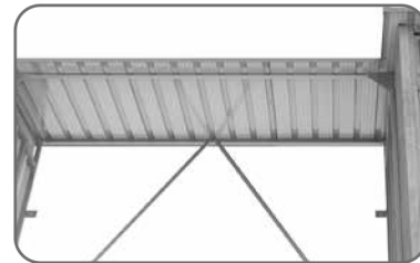
La fuerte armadura de acero del techo soporta 6,8 kgs./m2 de carga de nieve
