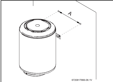
Fig. 9 Installazione verticale
