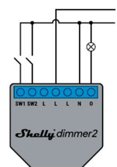
Cableado estándar con neutro y SW conectado al neutro
